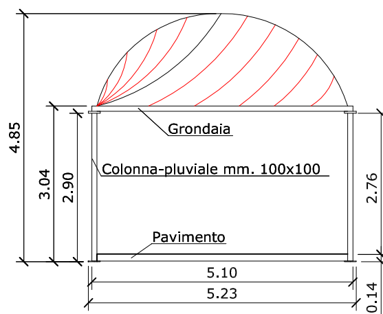
- PROSPETTO
